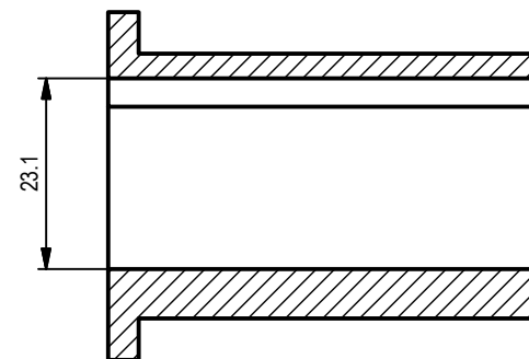
SECTION DM-DM SCALE 1 : 1
